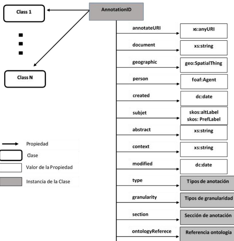
Fig. 4. Instancia de la clase AnnotationID (Fuente: elaboración propia)
